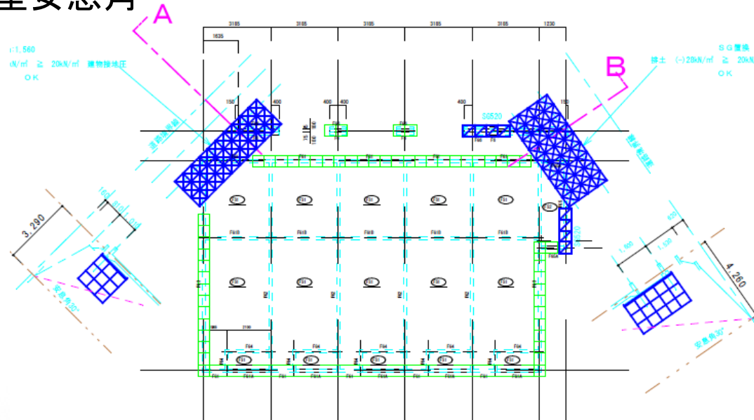
擁壁安息角
